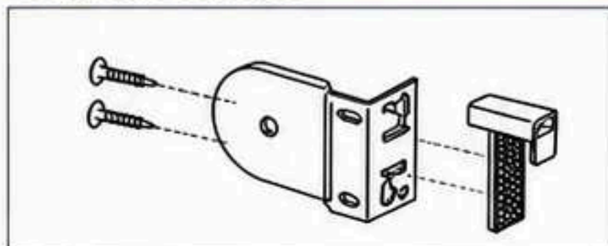
Atornillar
