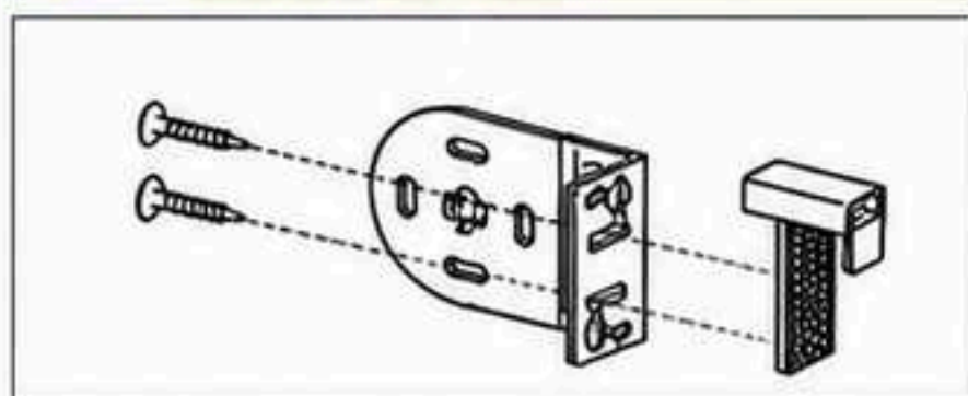
Atornillar
